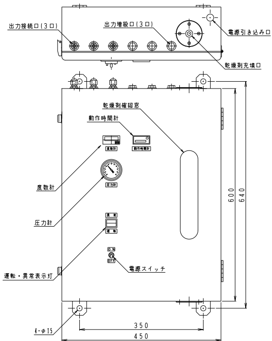
DHK-3(壁掛型)
