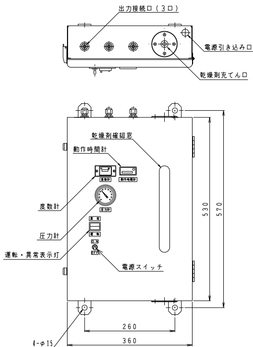
DHK-2(壁掛型)
